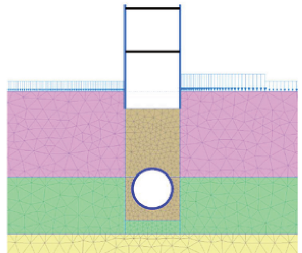
FEM Modellierung der Untergrundverhältnisse; Grafik: Ing. Büro LOGIC
