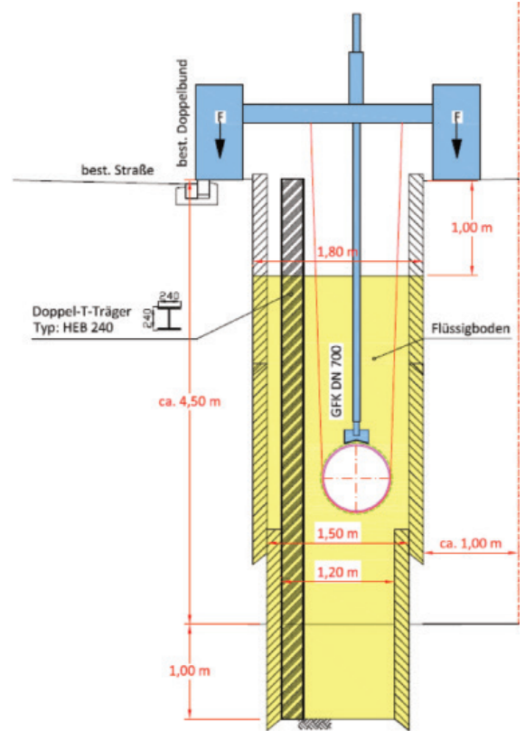
Weinfelden: Schnittzeichnung, Grafik: Ingenieurbüro LOGIC
