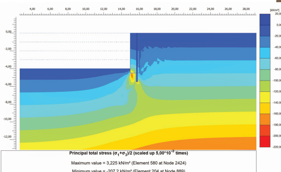
RSS Wand auf der Baustelle in Bad Rappenau - in der Phase des Endaushubs der Grube, d.h. der höchsten Belastung der RSS Wand - und das dazugehörige FEM-Modell zur Berechnung der Lastenverteilung. Foto + Grafik: Ingenieurbüro LOGIC
